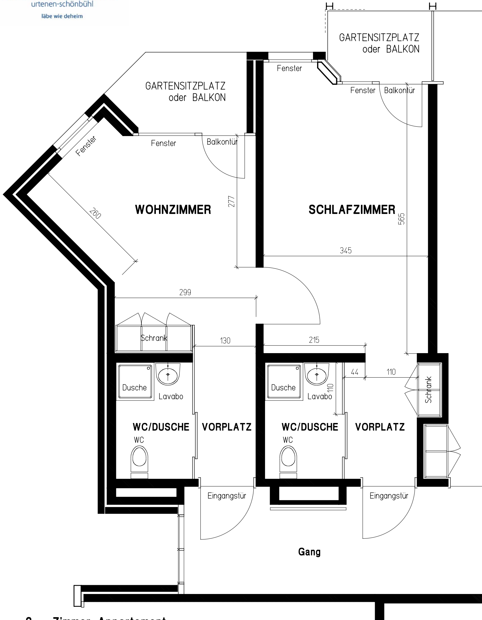
2 - Zimmer Appartement ZIMMERGRUNDRISS 1 : 50
